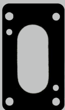
3-16-029 Baquelita Separador Carburador R-9 Corriente
