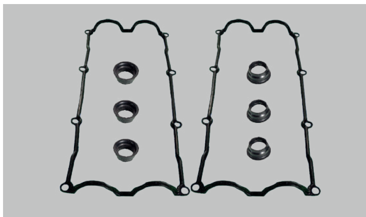
4-02-97172 Juego Empaquetaduras Tapa Válvula y Retenedores D - Max 3,5 CC
