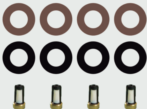
REF 4-20-30A KIA - BMW Con suministros de aire externo 4 inyectores microfiltros 6 mm oring en viton
