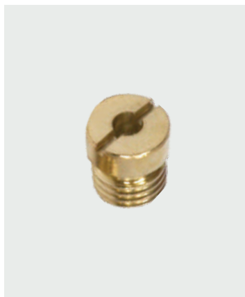
3-02-23 Chicler Alta N° 165
