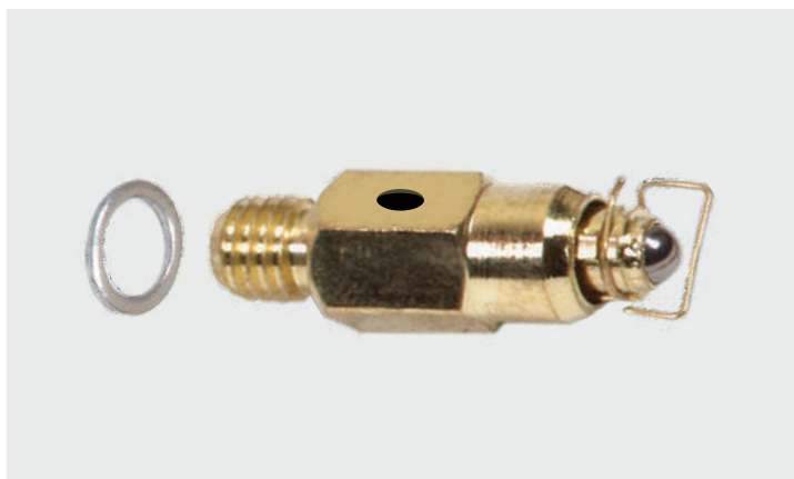
3-06-15 Base y Punzón Weber N° 175
