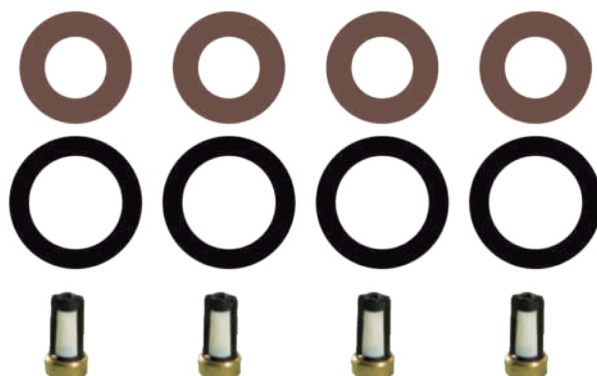
REF 4-20-31A DAEWOO Cielo, Lanos, Nubira, Tacuma, Leganza, Espero CHEVROLET Corsa, Cavalier, 2.2, Neon VOLKSWAGEN Vento FORD Fiesta 2001 KIA Sportage, 7-24, Cronos HYUNDAI Atos segunda serie 4 inyectores microfiltros 6 mm oring en viton UNIVERSAL
