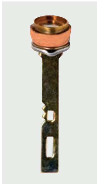
3-14-37 inyector Externo Paleta
