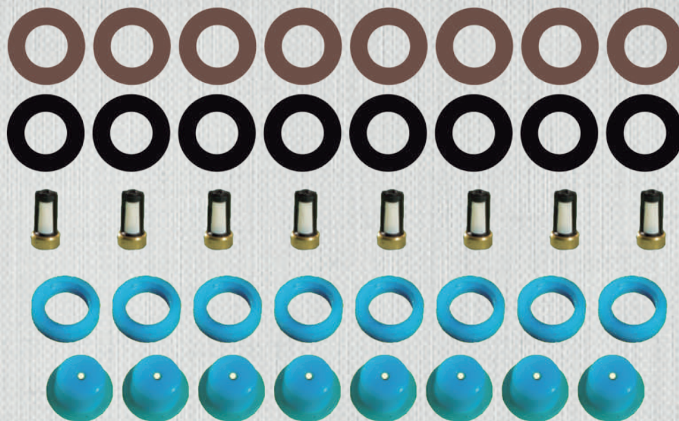
REF 4-20-15A FORD Bronco otros 8 inyectores microfiltros 6 mm oring en viton
