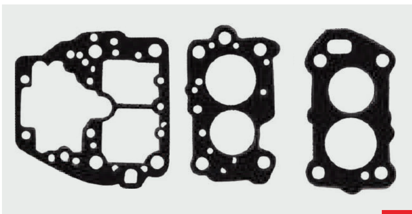
3-10-55 Juego de Empaques
