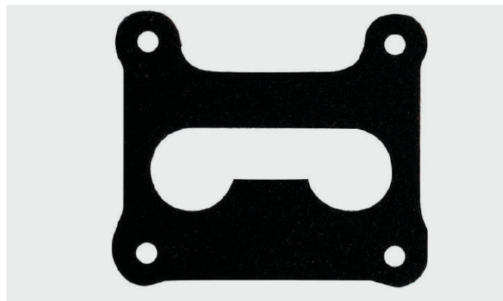
3-16-16 Baquelita Base Carburador
